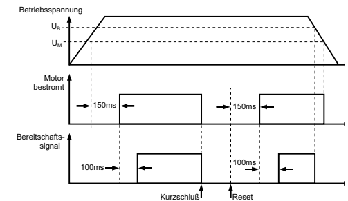
Abb. 5: Timing Bereitschaftssignal
