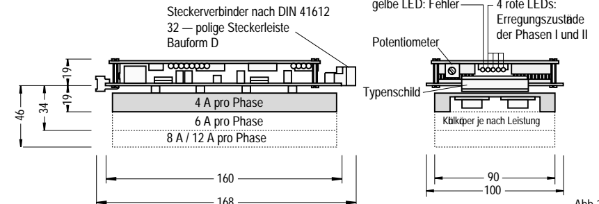
Abb.1: Abmaße
