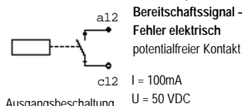
Abb. 4: Ausgangsbeschaltung
