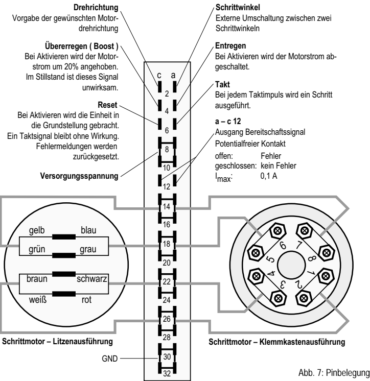
Abb. 7: Pinbelegung
